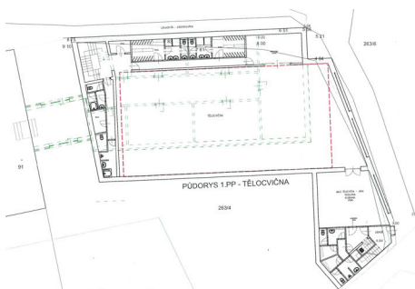
Půdorys prvního podlaží
